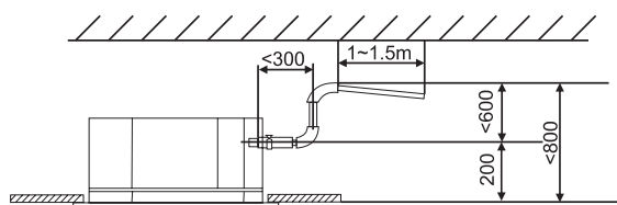
Рисунок 19 - Перегиб дренажной трубки
