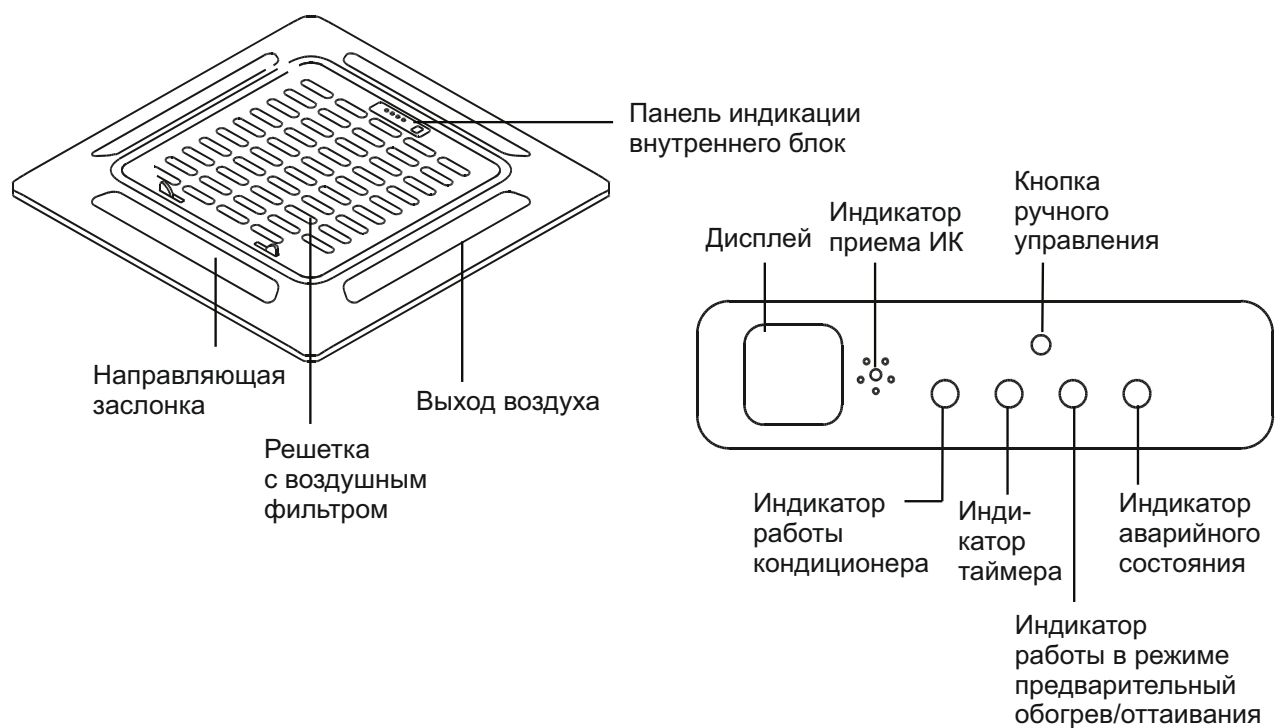
Рисунок 2.1- Панель индикации внутреннего блока кассетного типа
