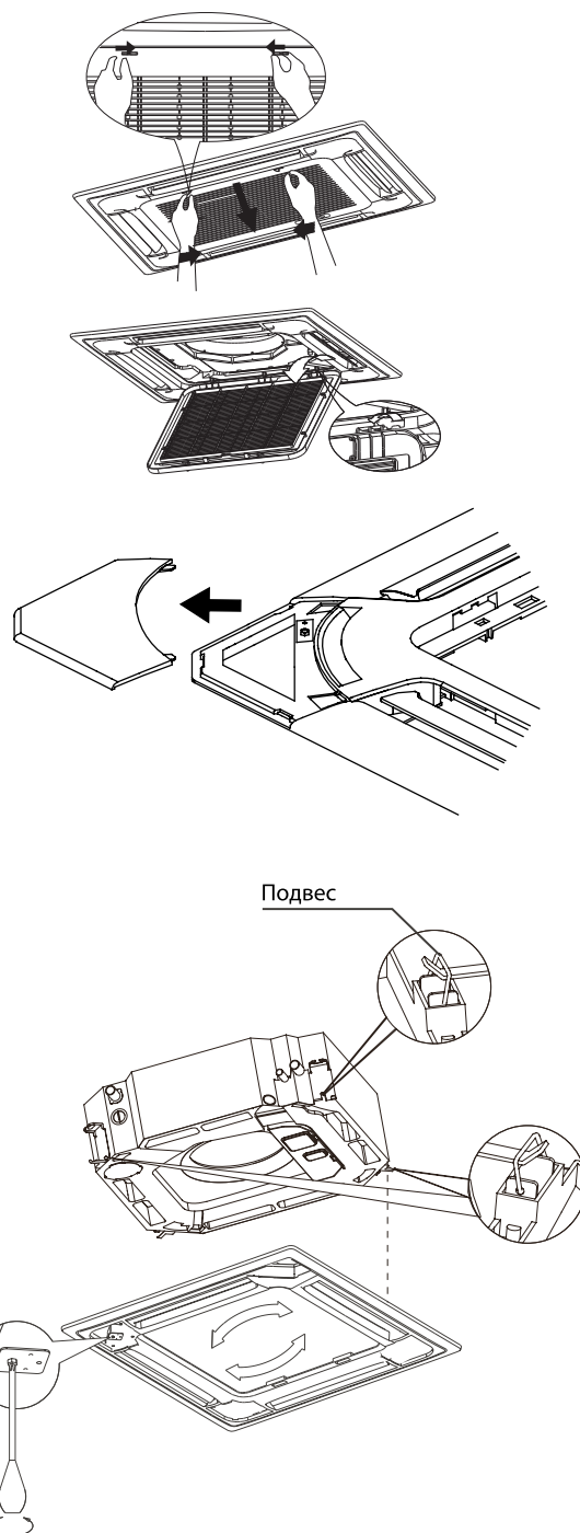
Рисунок 21 - Установка панели внутреннего блока
