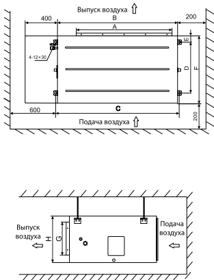
Размеры, мм.:
